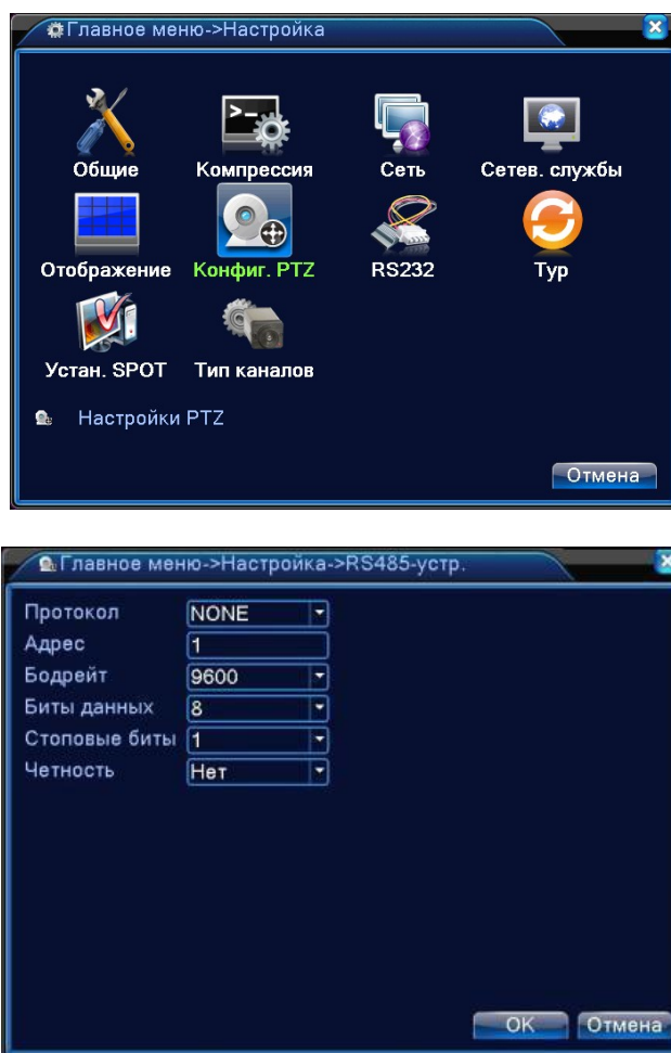
Рисунок 4.33 Конфигурация RS485 устройств в цифровом режиме.
