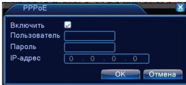
Рисунок 4.18 PPPoE
