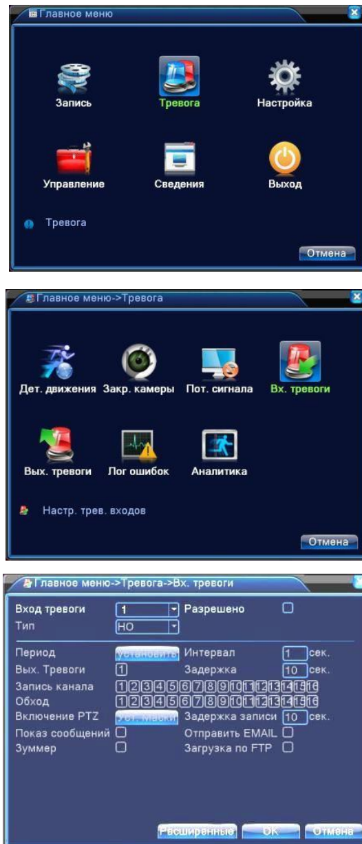
Рисунок 4.10 Вход Тревоги
