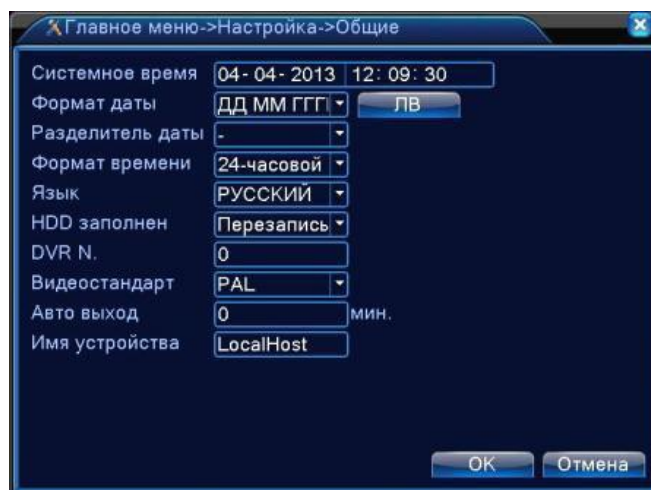
Рисунок 4.12 Общие настройки
