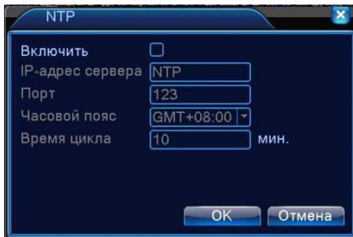
Рисунок 4.19 NTP
