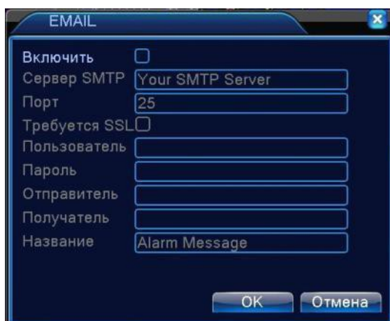
Рисунок 4.20 EMAIL
