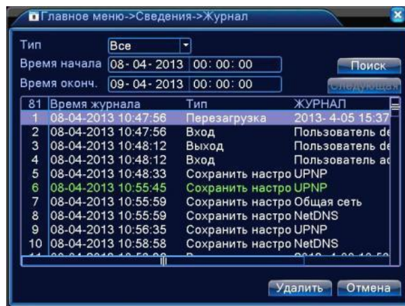
Рисунок 4.54 Информация журнала
