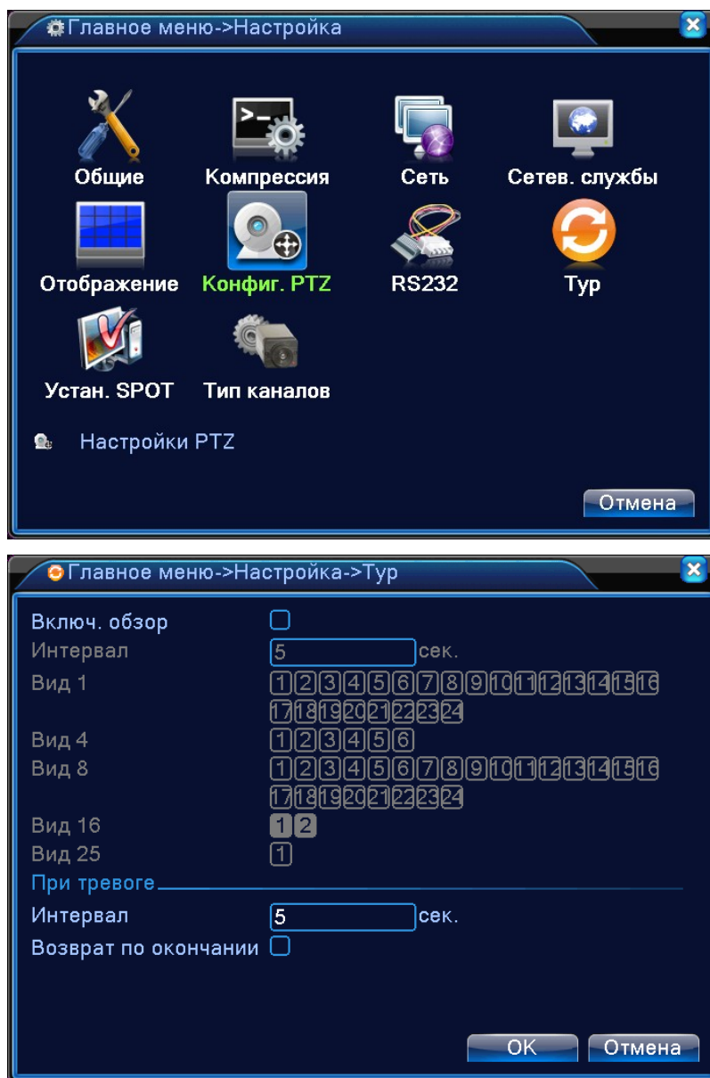
Рисунок 4.35 Настройка патрулирования
