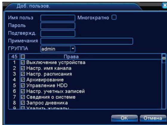
Рисунок 4.43 Добавить пользователя
