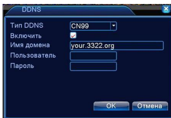
Рисунок 4.22 Настройки DDNS
