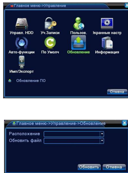
Рисунок 4.49 Обновление
