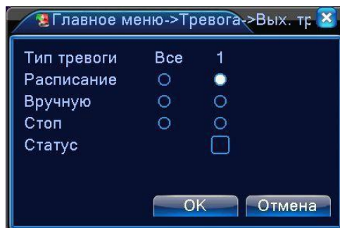
Рисунок 3.9 Тревожный выход
